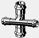
Prestabo-Križni kos s SC-Contur - jeklo nelegirano, pocinkano - stiskalni priključki Oprema Tesnilni elementi EPDM Model 1148
